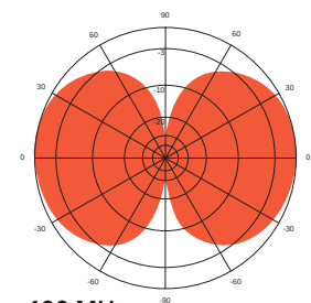
E-plane: 100 MHz
