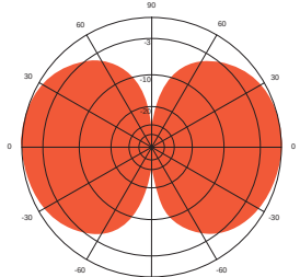
E-plane: 136 MHz
