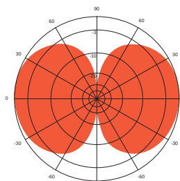
E-plane: 100 MHz
