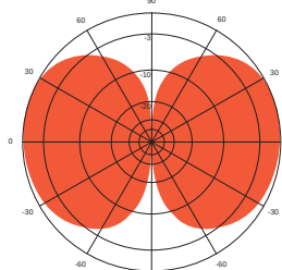
E-plane: 400 MHz
