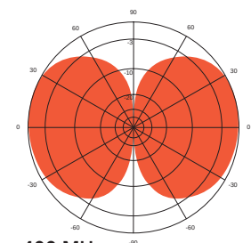
E-plane: 400 MHz
