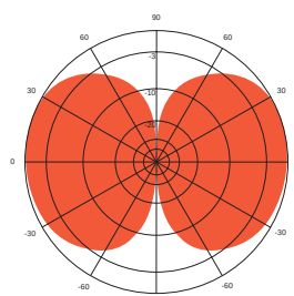
E-plane: 450 MHz
