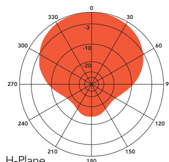
H-Plane Gain: 5.1 dBd
